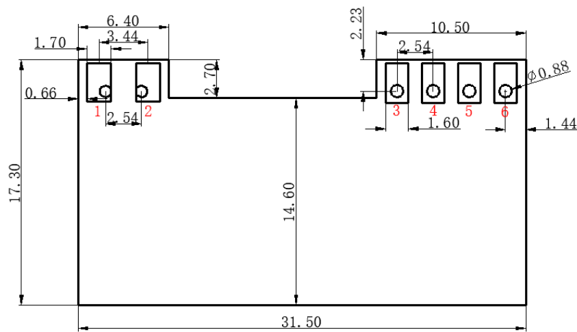
图 3 模块尺寸图
